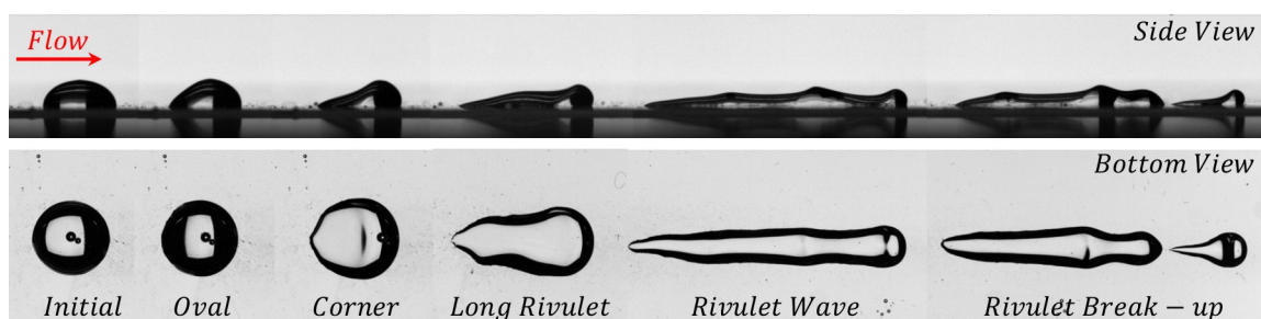
Fig. 1 : Exemple de visualisation de la dynamique d'une goutte mise en mouvement par un écoulement d'air sur une paroi plane (Chahine, PhD, 2023)
